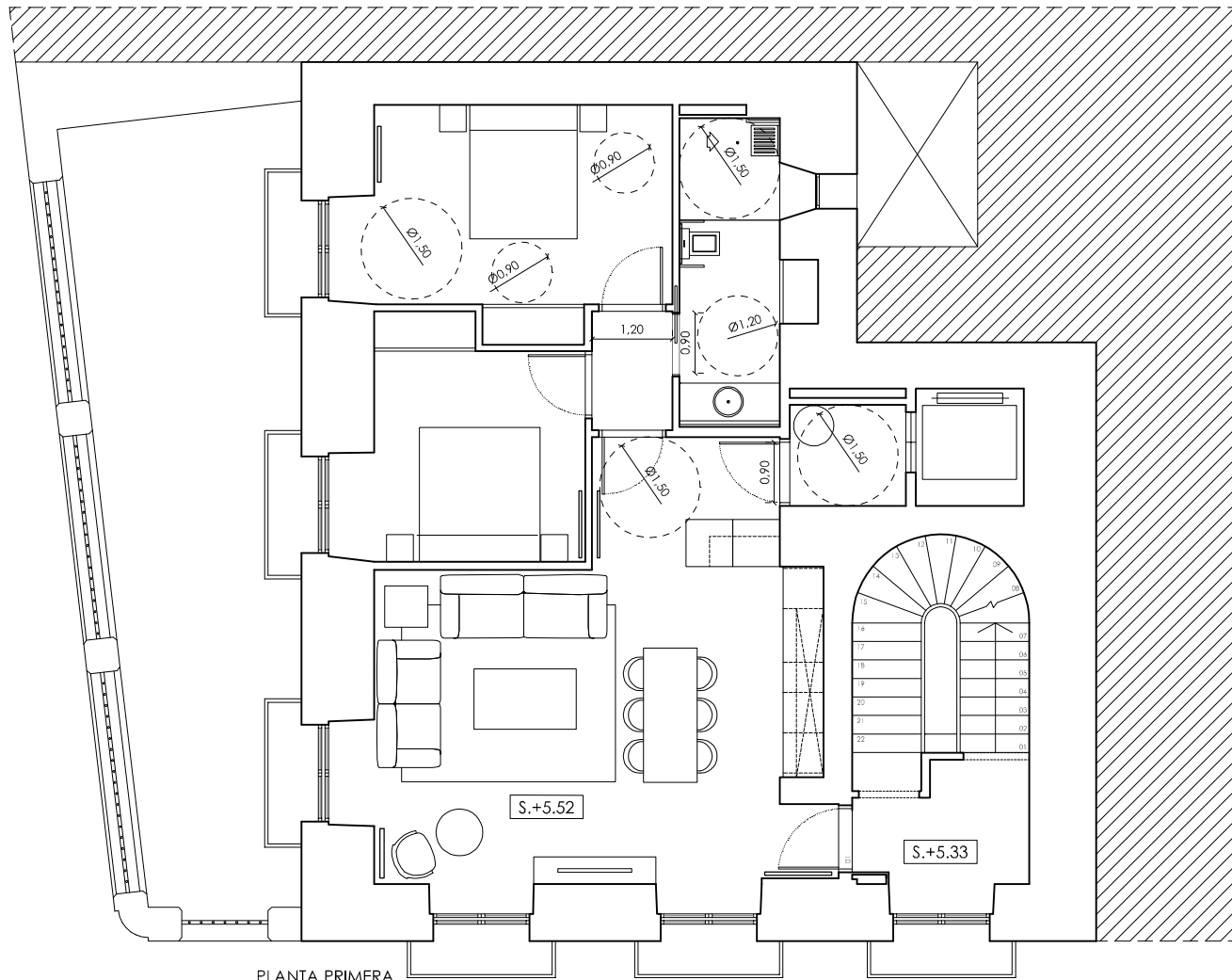
PLANTA PRIMERA
